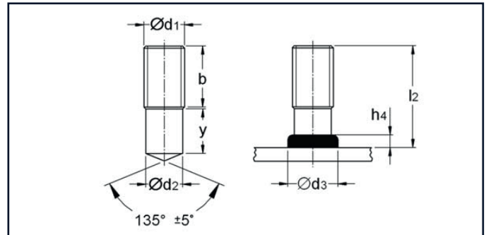
Threaded stud RD, dimensions acc. to EN ISO 13918
