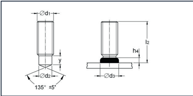
Gewindebolzen PD, Maße nach DIN EN ISO 13918
