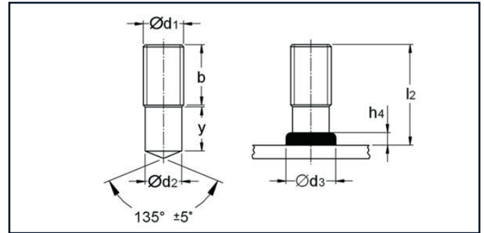
Gewindebolzen RD, Maße nach DIN EN ISO 13918
